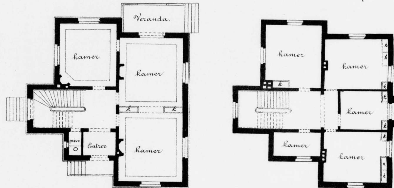
Bovenverdieping.
